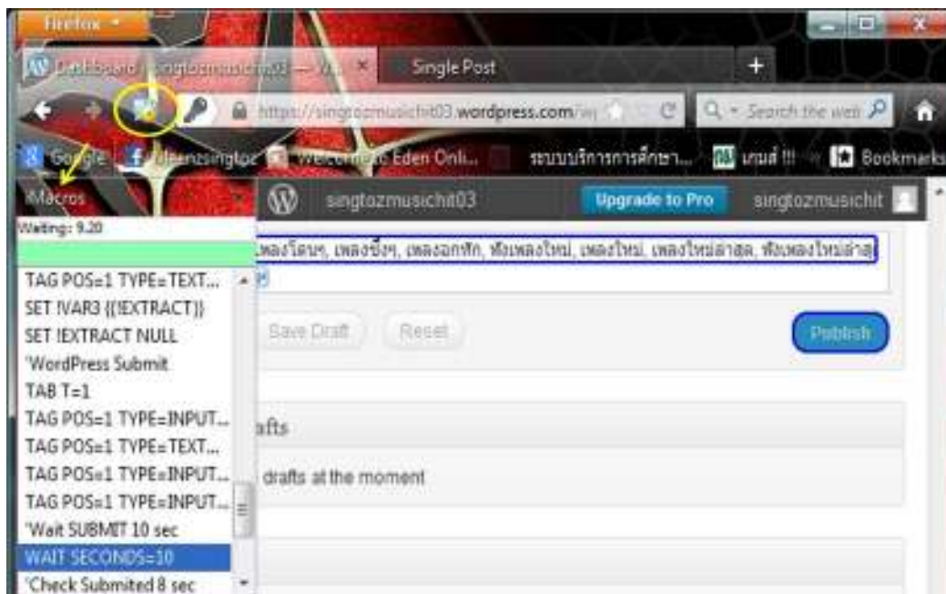
ตัวอย่าง การทำงานบางส่วนของโปรแกรม iMacros
